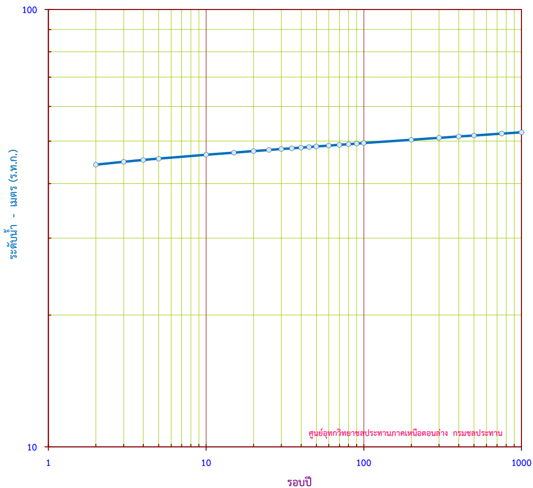
กราฟแสดง ระดับน้ำสูงสุดรายปี ขนาดรอบปีต่างๆ สถานี P.16 อ.ขามเฒ่า จ.กำแพงเพชร
